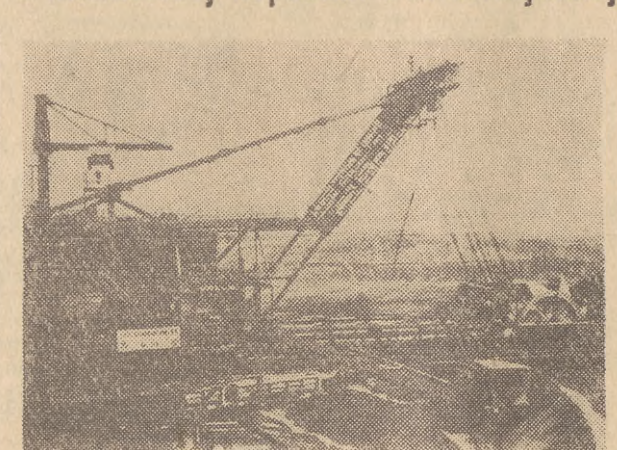
W kopalni odkrywkowej „Freundschaft” w Kletwitz pracuje olbrzymia koparka „Sch R 1000”, wyprodukowana w Zakładach Budowy Maszyn „Leuchhammerwerk”. Koparka napędziana łańcuchem 11-13 minut 8 specjalnych wagonów o pojemności 40 m sześciu, każdy. Fot. — CAF
