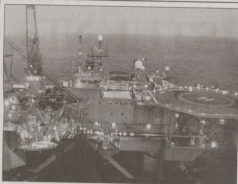
Regalia, norweski statek-platforma zakotwiczony na Morzu Barentsa w miejscu gdzie 12 sierpnia zatonił rosyjski atomowy okręt podwodny „Kursk”. Norweski statek-platforma, uczestniczy w akcji wydobywania zwłok z wraku rosyjskiego okrętu atomowego.
