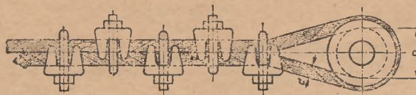
bei d=10\text{ mm} D mindestens 3d bei d=50\text{ mm} D mindestens 4d für Zwischenwerte d geradlinig einschalten
