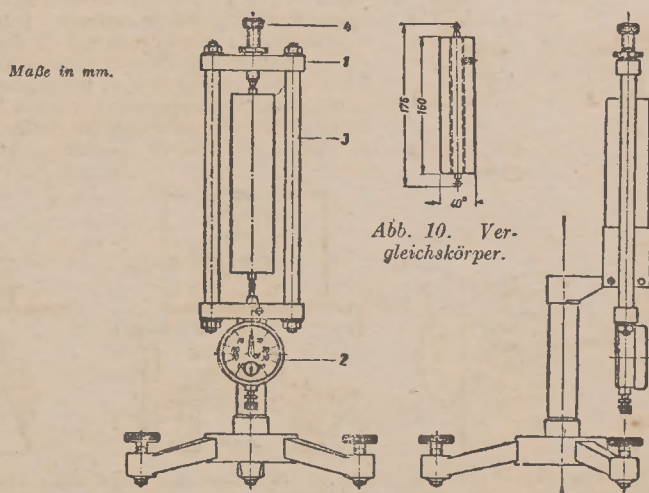
Abb. 9. Schwindmeßgerät.
