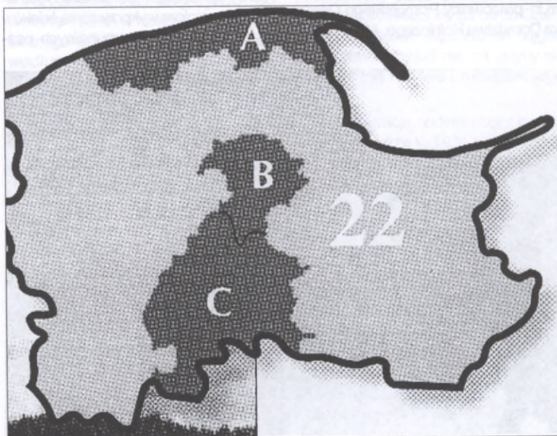
Strefy priorytetowe woj. pomorskiego: A – półwyspy Słowińskiego i Gdańskiego, B – centralna pojezierza, C – Borów Tucholskich i Równiny Charzykowskiej
