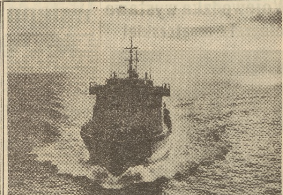
Próbny rejs nowego wielkiego lodolamacza fińskiego „Varma" o wyporności 5000 ton, długości 86,5 m i szerokości 21,2 m. W związku ze specjalnymi zadaniami jakie stoją przed lodolamaczami, poddaje się je pięciu próbom, podczas gdy zwykły frachtowiec przechodzi tylko jedną. CAF — Leht
