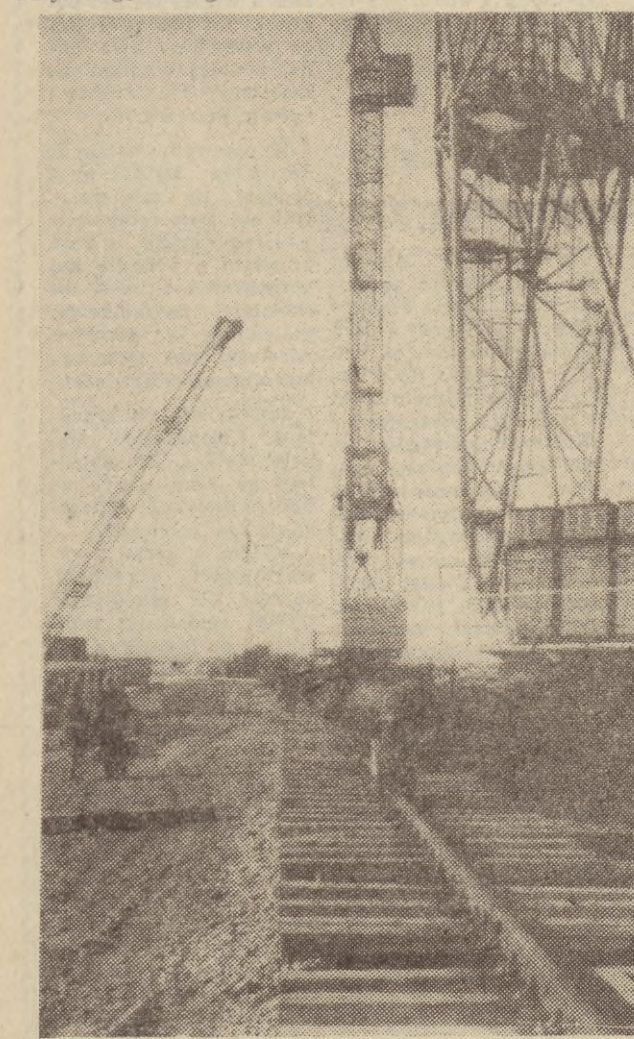
Na zdjęciu zmontowane dźwigi — żurawie radzieckie o udźwigu 160 ton metrow.
