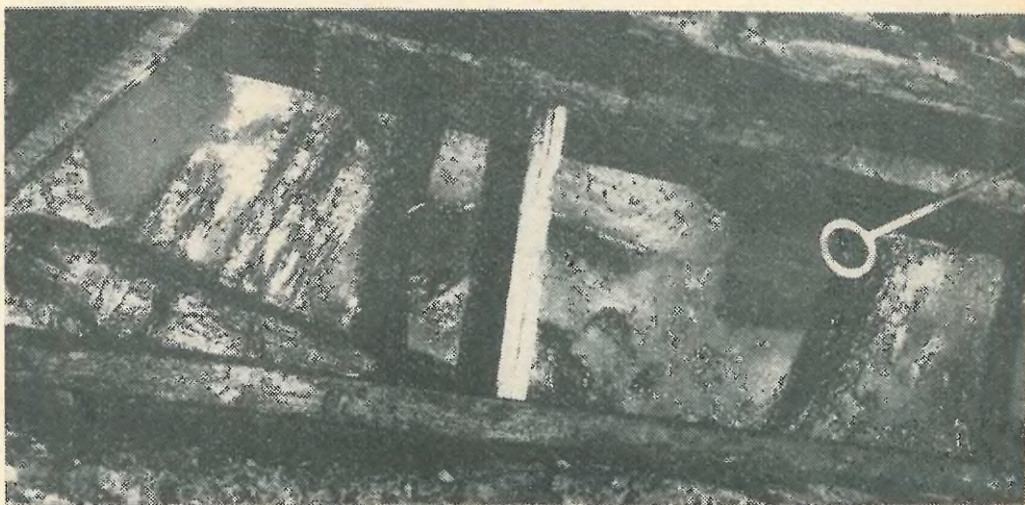
WYKOP I. NA DNIIE WYKOPU WIDOCZNE FRAGMENTY LEGARÓW ULICZNYCH PRAWDOPODOBNIIE Z LAT 1261—1263 (?)
