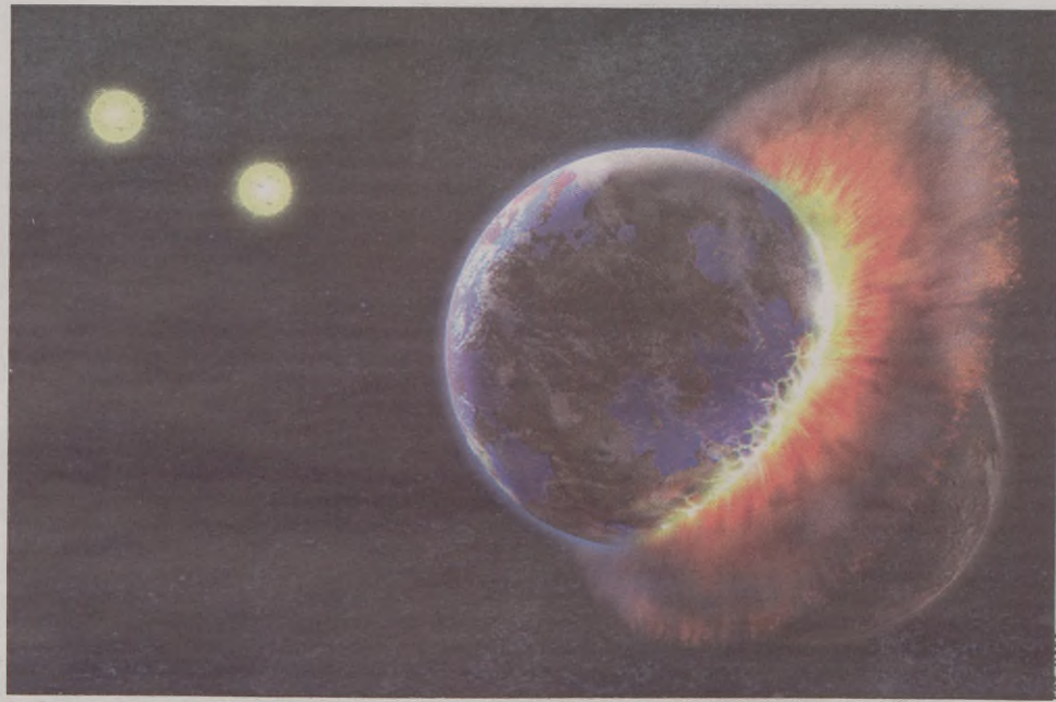
Tak mogło – według naukowców – wyglądać zderzenie planet.
