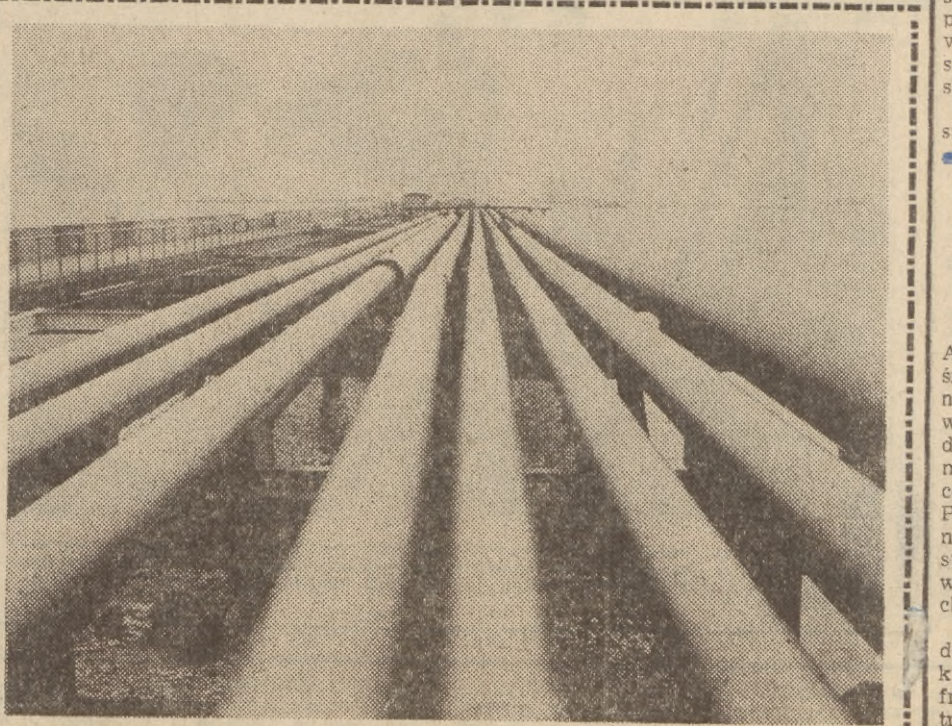
Port Północny — rurociągi przy pirsie paliw płynnych. Fot. W. Nieżywiński
