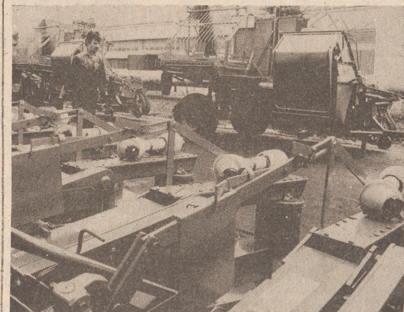
Kosiarki rotacyjne i kombajny do zbioru buraków cukrowych stanowią podstawę produkcji słupskiego „Famarolu”, a także są przedmiotami sprzedaży dla krajowych i zagranicznych odbiorców.
