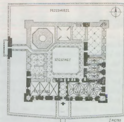
Radzyń Chełmiński. Plan zamku
