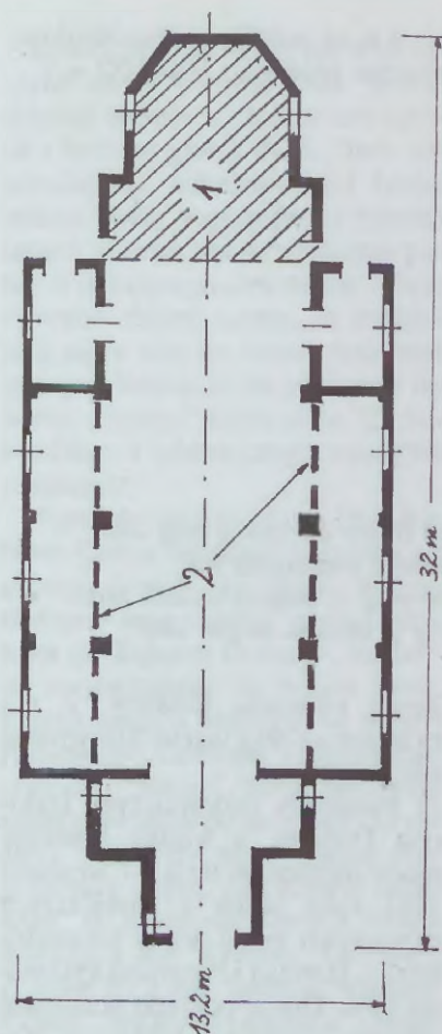
Rzut poziomy kościoła w Tyłowie: 1 - prezbiterium i część nawy dawnego kościoła, 2 - nie wykonana propozycja wewnętrznych ścian konstrukcji szkieletowej
