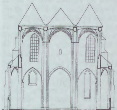
Kościół św. Jana w Toruniu. Przekrój poprzeczny
