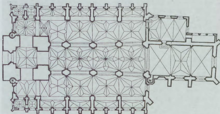
Rzut kościoła św. Jana w Toruniu wg Heisego
