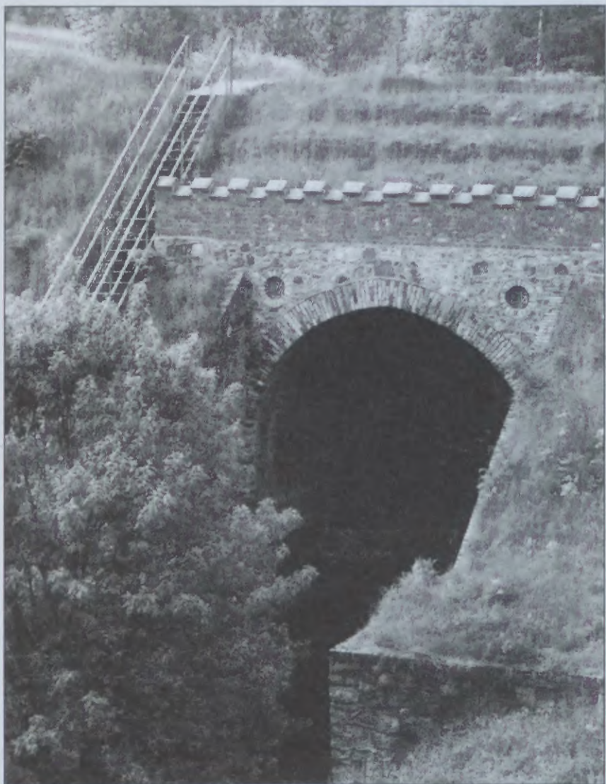
Akwedukt w Fojutowie (1848 r.)
