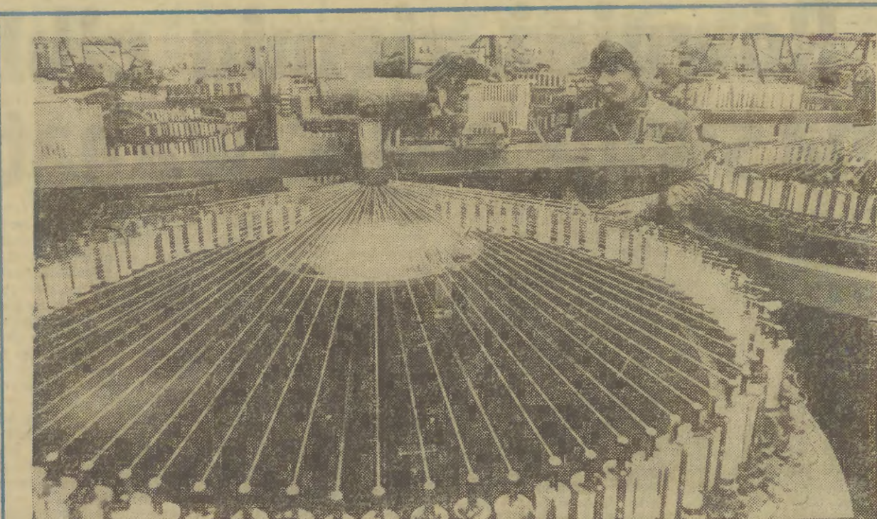
W związku z brakiem bawelny z importu Zakład Koronkarski w Brzozowie, wchodzący w skład Fabryki Furanek w Skopaniu, przeznaczając swoją produkcję głównie na pokrycie zapotrzebowania wynikającego z programów operacyjnych, dla złagodzenia trudności surowcowych część koronek wytwarza się z elastanu. Uruchomiono również produkcję nici obuwniczych i plecionek do szycia mokraków.
