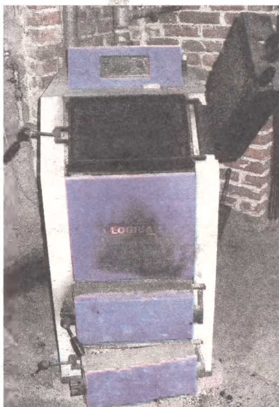
Współczesne kotły na paliwo stałe wyposażone są najczęściej w sterowniki, które umożliwiają nastawienie parametrów pracy. Dzięki temu proces spalania jest bardziej ekonomiczny. Fot. mk
