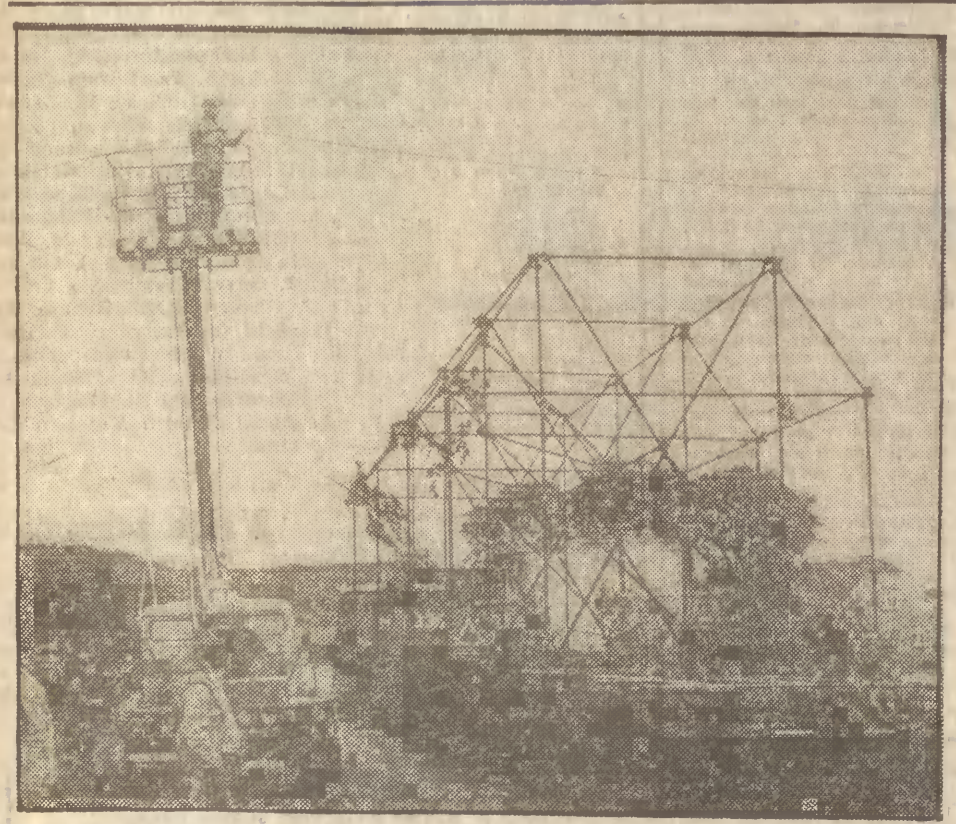
Zakład Transportu Energetyki Radom na polecenie Elektrowni Jadrowej „Zarnowiec” podjął się przewiezienia reaktora z Portu Gdynia do Zarnowca (trasa 70 km w III kw. 1988 r.). Obecnie przeprowadzono próbe transportu makiety reaktora na platformie 120-kolowej trasie przyszłego przejazdu reaktora Gdynia — Reda — Puck Zarnowiec. Przejazdem i służbą drogową kieruje inż. Edward Dąbrowski z Elektrowni Jadrowej „Zarnowiec”. N.Z.: przejazd platformy z makieta na trasie w Rumli. CAF telefona Janusz Uklejewski
