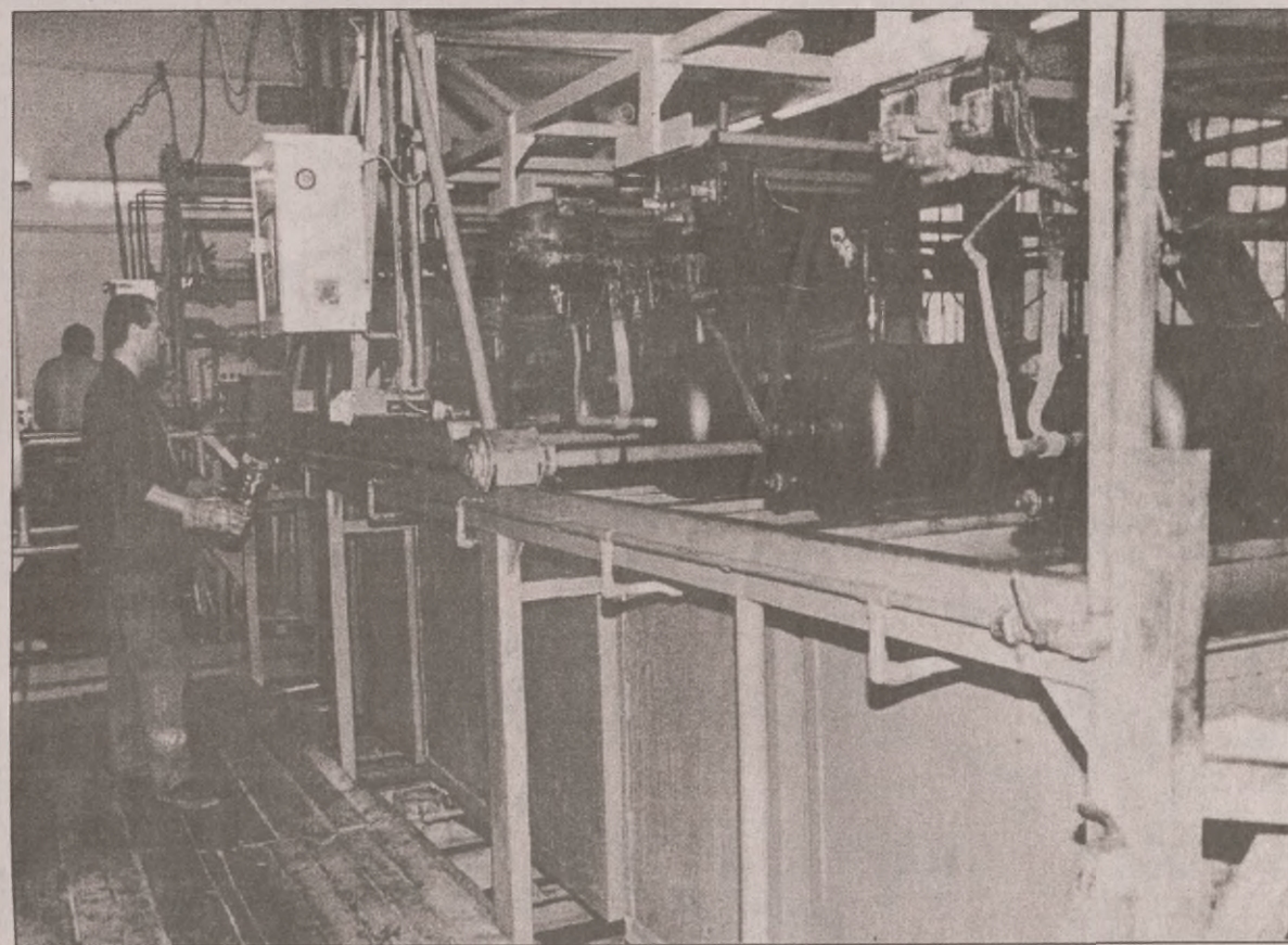
Po próbach ciśnieniowych bojlery trafiają do kadzi, gdzie są pokrywane antykorozyjną substancją.
