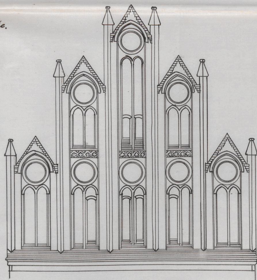
Ansicht des Ostgiebels.
