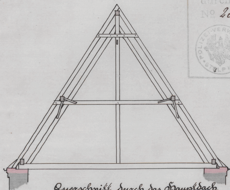
Querschnitt durch das Hauptdach.
