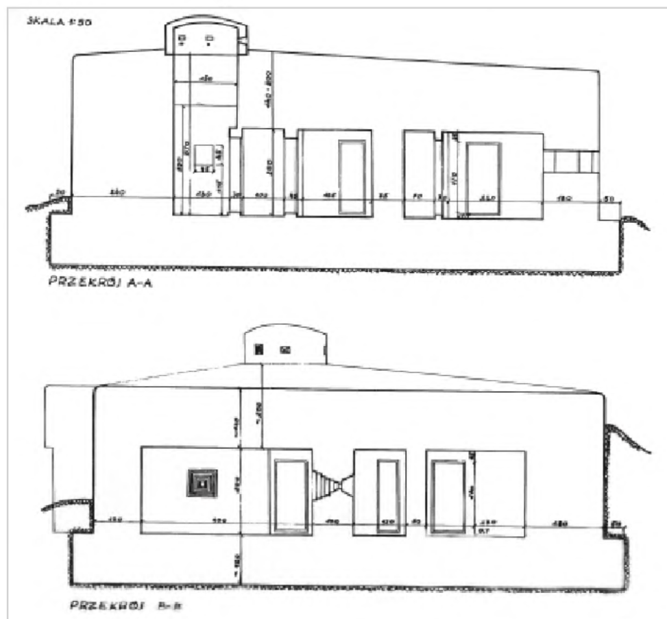
Przekrój obiektu Nr 10214 - X-II
