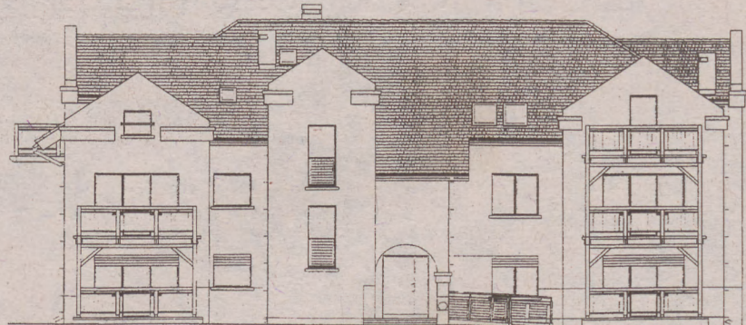
elewacja frontowa
