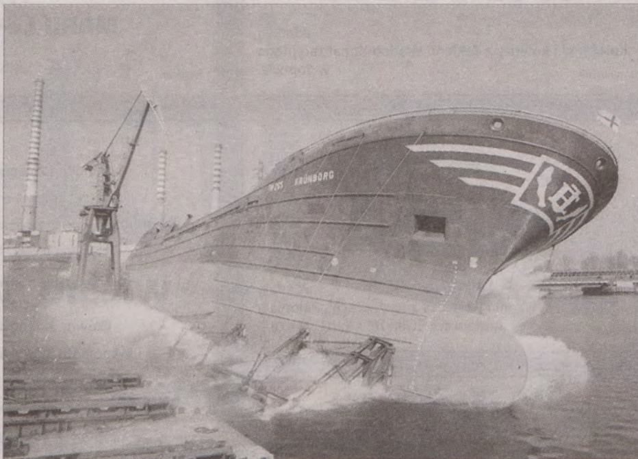
Z pochylni bocznej Stoczni Północnej w Gdańsku zwodowano kadłub statku rybackiego „Krunborg” dla kontrahenta z Norwegii.
