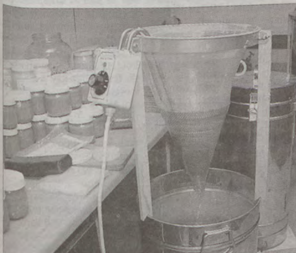
Urządzenie do „gorącego” odwirowywania miodu z plastrów.
