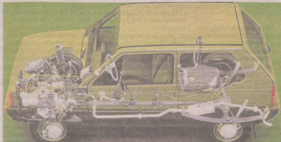
„Rentgenowski” rysunek pozwala ocenić prostotę układu napędowego. Tyłne resory odmiany 4x4 miały trzy pióra. W zwykłej Pandzie - jedno
