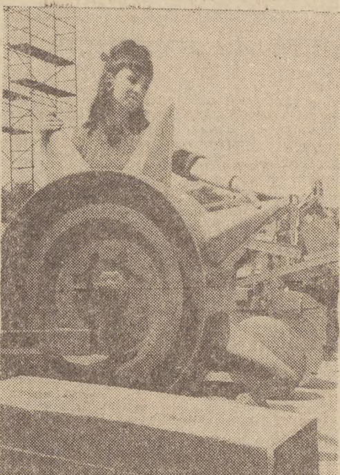
Na zdjęciu po lewej — „kolczatka” — urządzenie mechaniczne do sadzenia lasu, wyprodukowane przez warsztaty OZLP w Szczecinku. Niżej — samojedźny dźwąg i podnośnik — produkowane przez Fabrykę Urządzeń Budowlanych w Koszalinie. Fot. J. Piątkowski
