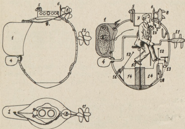
Rys. 1. „Żółw” Buschenella. 1 — mina, 2 — ciężar denny nadający stateczność, 3 — mechanizm zegarowy miny, 4 — ster, 5 — odwietrzniki, 6 — linka łącząca minę ze świderem, 7 — wieżyczka, 8 — śruba pionowa, 9 — śruba pozioma, 12 — pompy do balastu wodnego, 13 — kingston do napełniania komór balastowych wodą, 14 — komory balastowe, 15 — urządzenie do odczepiania ciężaru dennego, 16 — otwory pomp balastowych
