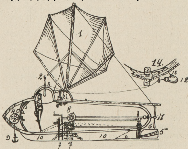
Rys. 2. „iNautle” Fultona. 1 — żagle, 2 — świder, 3 — luka wejściowa, 4 — dźwig kotwiczny, 5 — ster poziomy, 6 — ster pionowy, 7 — pompy, 8 — mechanizm śruby napędowej, 9 — kotwica, 10 — komory balastowe, 11 — śruba napędowa, 12 — mina, 13 — zapalnik miny, 14 — część podwodna okrętu atakowanego
