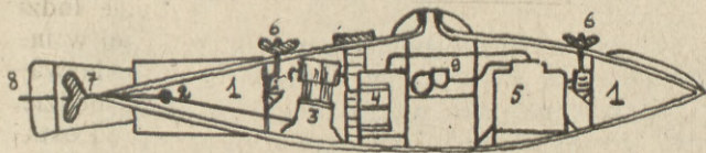
Rys. 6. Łódź (podwodna Nordenfelda. 1 — komory (balastowe, 2 — krzyżulec, 3 — maszyna parowa, 4 — komora parowa, 5 — zbiornik do magazynowania pary, 6 — śruby pionowe, 7 — śruba napędowa, 8 — ster, 9 — postereunek centralny
