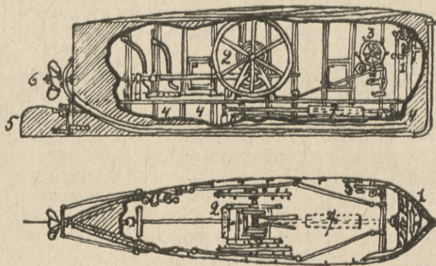
Rys. 3. „Diabeł morski” Bauera. 1 — dźwign kotwiczna, 2 — mechanizm śruby napędowej, 3 — pompa, 4 — komory balastowe, 5 — eter, 6 — śruba napędowa, 7 — ciężar przenośny
