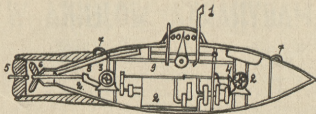
Rys. 7. Łódź podwodna Inż. Drzewieckiego. 1 — peryskop, 2 — komory balastowe, 3 — silnik elektryczny, 4 — pumpy, 5 — stery poziome i planowe, 6 — śruba napędowa, 7 — uchwyty do podnoszenia łodzi, 8 — krzyżulec, 9 — postereunek centralny
