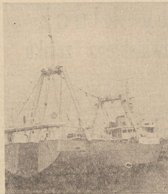
Stocznia im. Komuny Paryskiej w Gdyni przekazała armatorowi islandzkiemu drugi z kolei trawler rybacki typu B-425 m/t „Ogri”. Pierwszy — m/t „Vigri”, płynący od kilku miesięcy pod banderą Islandii — pełni rolę statku flagowego floty rybackiej tego kraju „Centromor” podjął z armatorem islandzkim kontrakty na budowę siedmiu statków tego typu. Na zdjęciu: m/t „Ogri” w basenie „Komuny” przed wypłynięciem do Islandii.
