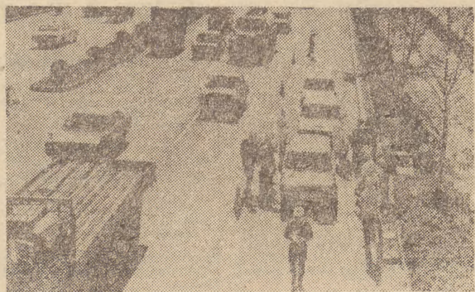
Ostatnio policja japońska przeprowadziła w prefekturze Tokio badania zawartości tlenku węgla w spalalinach samochodów. Jeśli za wartość CO przekraczała 4,5 proc., właściciel pojazdu musiał zapłacić grzywnę w wysokości 10–20 dolarów USA.
