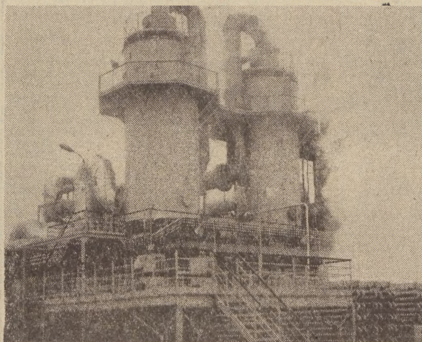
W Zakładach Azotowych w Puławach uruchomiono pierwszy węzł technologiczny wytwórni kwasu siarkowego i oleum — jednego z surowców do produkcji włókien syntetycznych. Po wybudowaniu instalacji kaprolaktanu — stanie się jego baza surowcowa. %alkowite zakończenie prac związanych z wznoszeniem wytwórni nastąpi za dwa lata. Na odjęciu: nowa wytwórnia kwasu siarkowego w Puławach.
