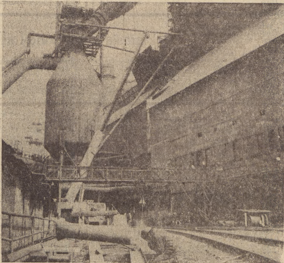
Największy piec Huty im. Lenina którego pojemność wynosi 2002 m sześciennie, przechodzi obecnie cyklowny remont. Początkowo zakładany okres remontu miał wynieść 56 dni, jednak ze względu na ciągłe zanotowanie na stal skrócono czas naprawy do 44 dni. Zastosowano nowy sposób spawania wymienianego kadłuba stalowego z elementami scalonymi. Inne nowości to zastosowanie dźwigów samojedźnych. Na zdjęciu: widok remontowanego pieca.
