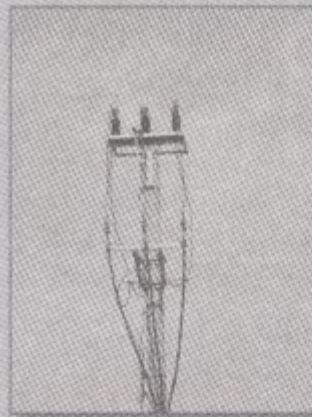
Конструкция под ограничители перенапряжений
