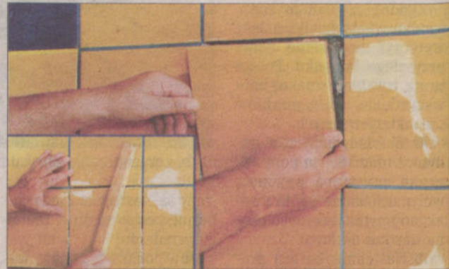
Wstawiamy płytkę, przykładamy do niej listwę lub poziomnicę i całość dociskamy do podłoża, tak aby zrównać powierzchnie płytki i całej okładziny. Po 48 godz. uzupełniamy brakującą fugę.
