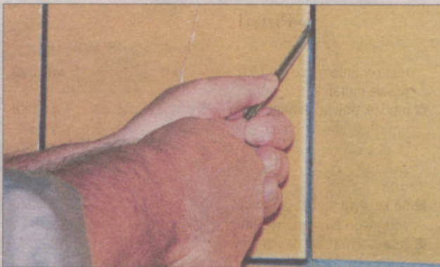
Odkucie pękniętej płytki wiąże się z ryzykiem uszkodzenia sąsiednich. Aby tego uniknąć, trzeba usunąć starą fugę wokół zniszczonej płytki, używając w tym celu specjalnego rylca lub przecinaka.
